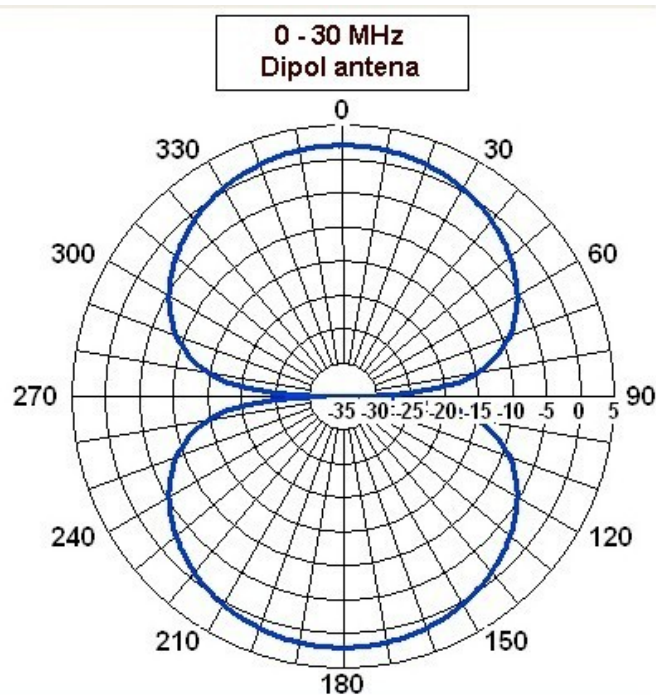
Horizontalni dijagram zračenja
