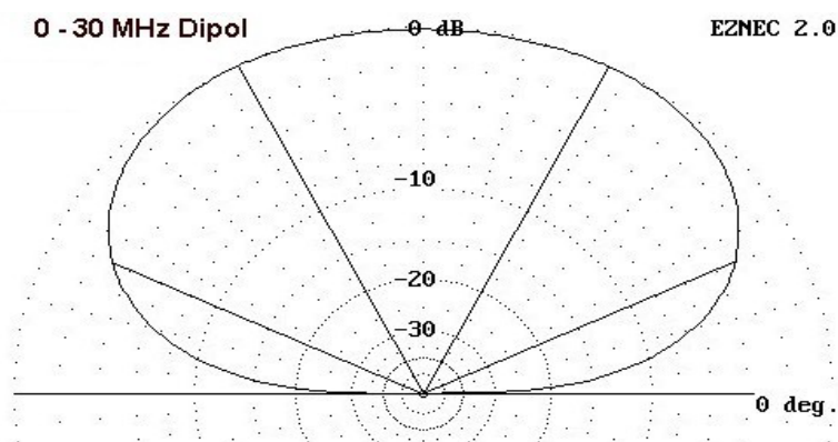
Vertikalni dijagram zračenja
